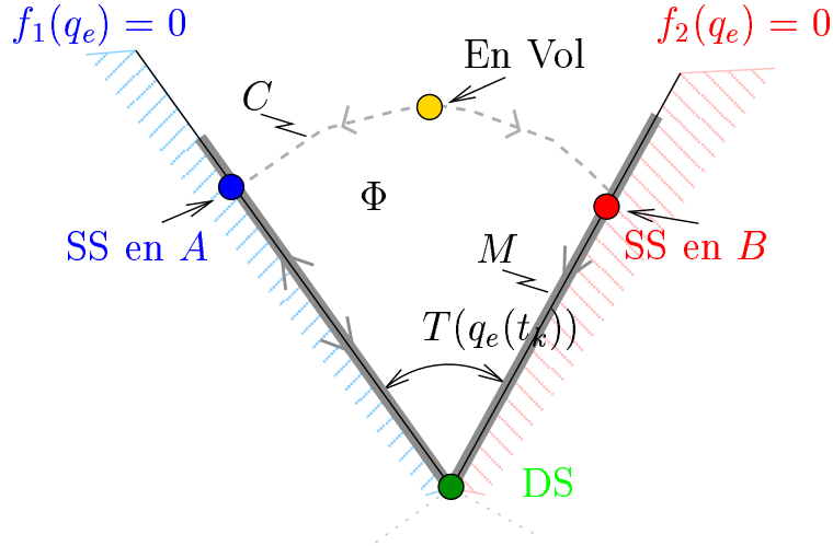
FIG. 8.6 – Contraintes dans l'espace des coordonnées généralisées
