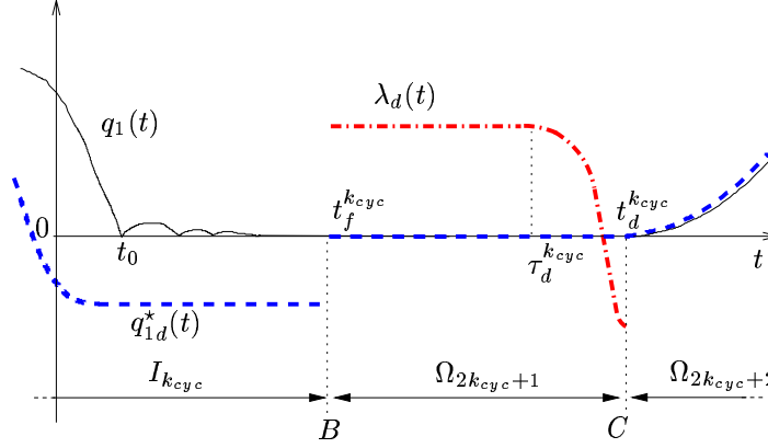
FIG. 4.4 – Trajectoire désirée de \lambda_d
