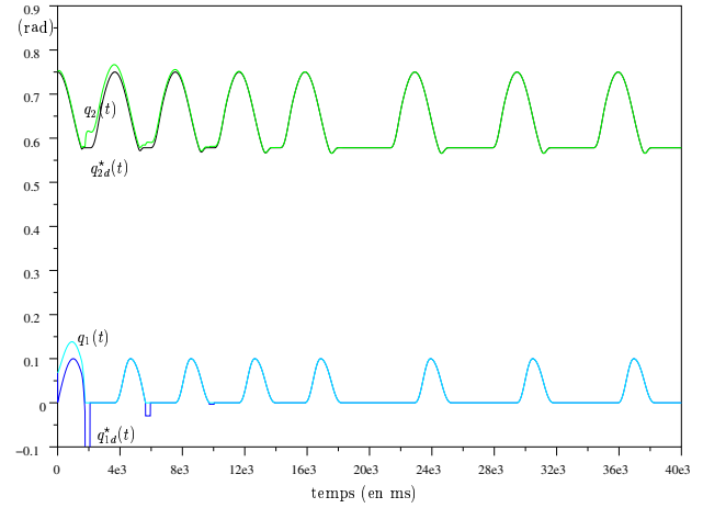
FIG. 6.14 – n° 7: q_d^*(t) et q(t) pour \alpha = 0 FIG. 6.15 – n° 8: q_d^*(t) et q(t) pour \alpha = 100
